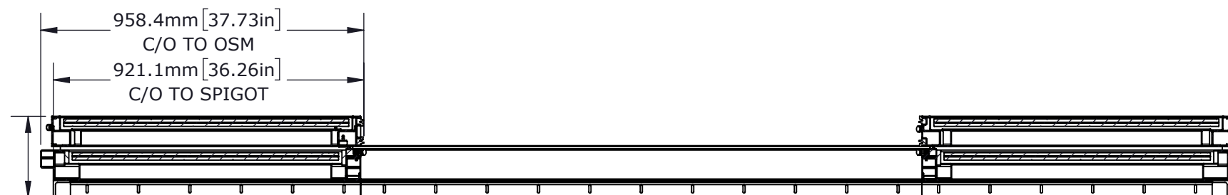
SECTION A-A SCALE 1 : 16
